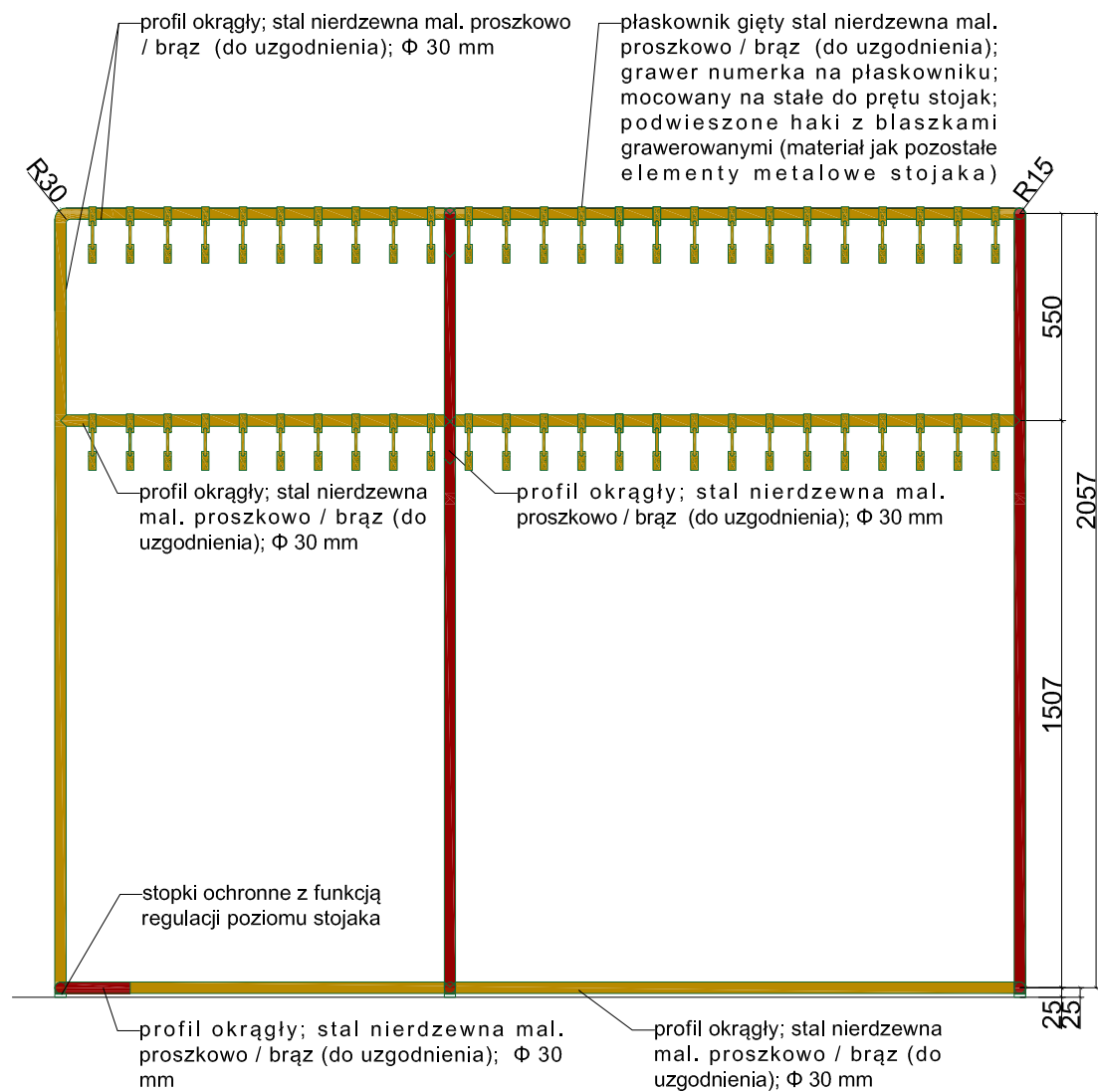
WIDOK A
