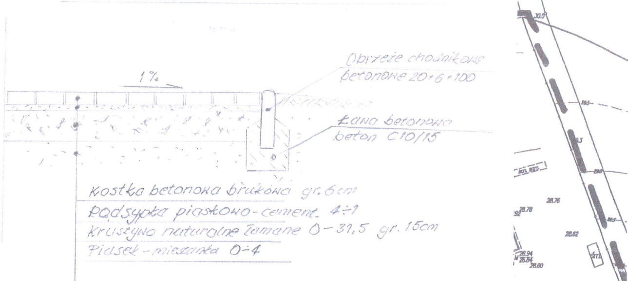
PRZEKRÓJ PŁACU I CHODNIKA
