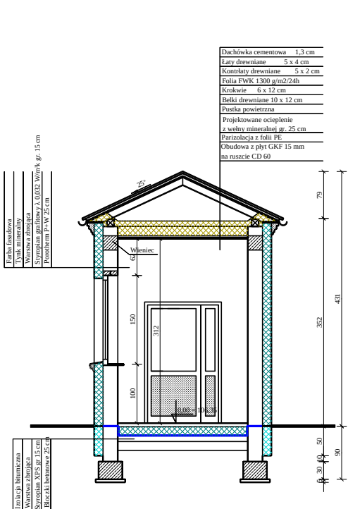
PRZEKRÓJ PIONOWY II - II
