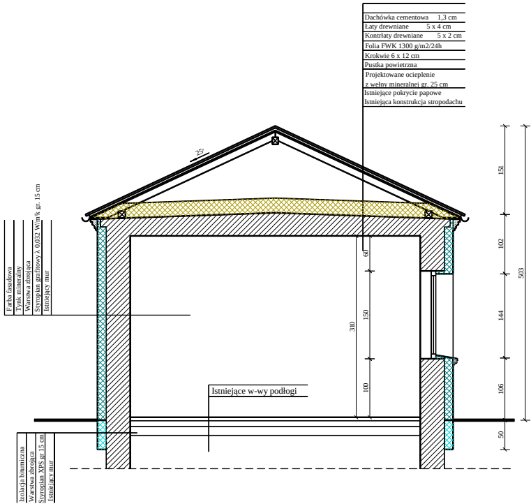
PRZEKRÓJ PIONOWY I - I
