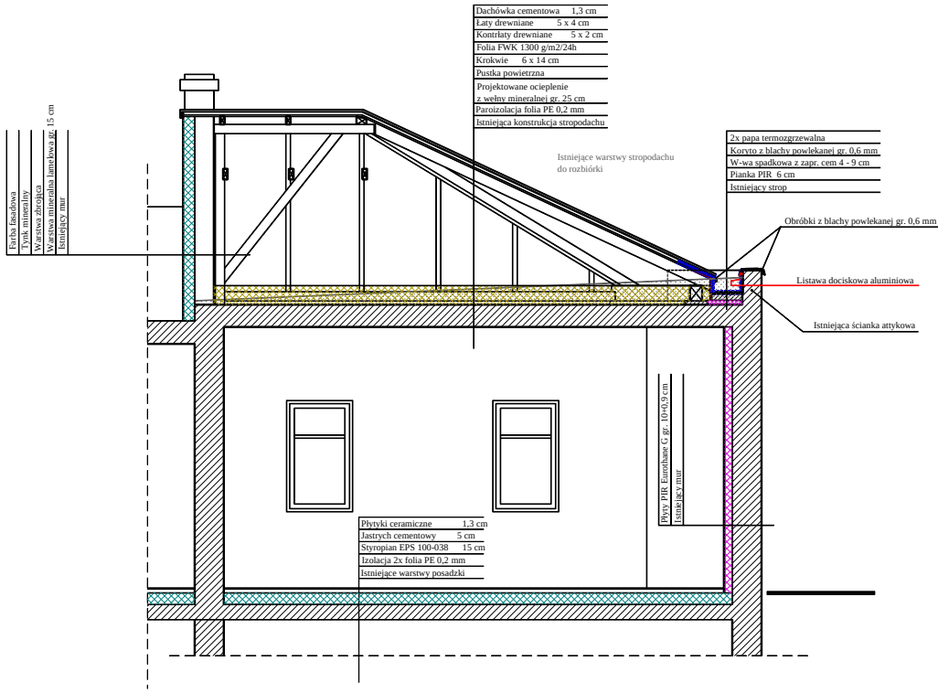
PRZEKRÓJ PIONOWY III - III
