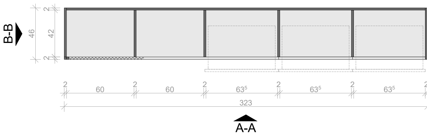
przekrój poziomy 1-1
