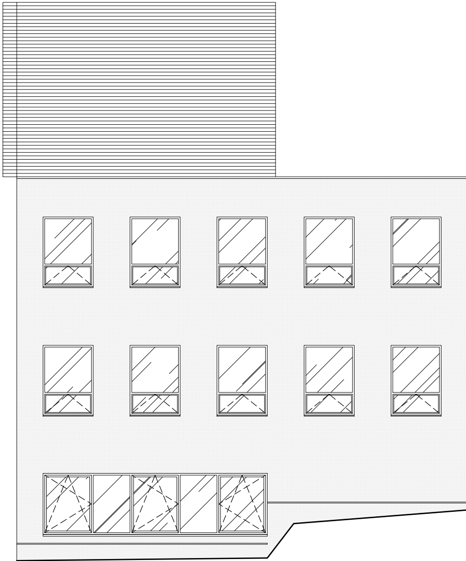
ELEWACJA PÓŁNOCNO - ZACHODNIA (PATIO)
