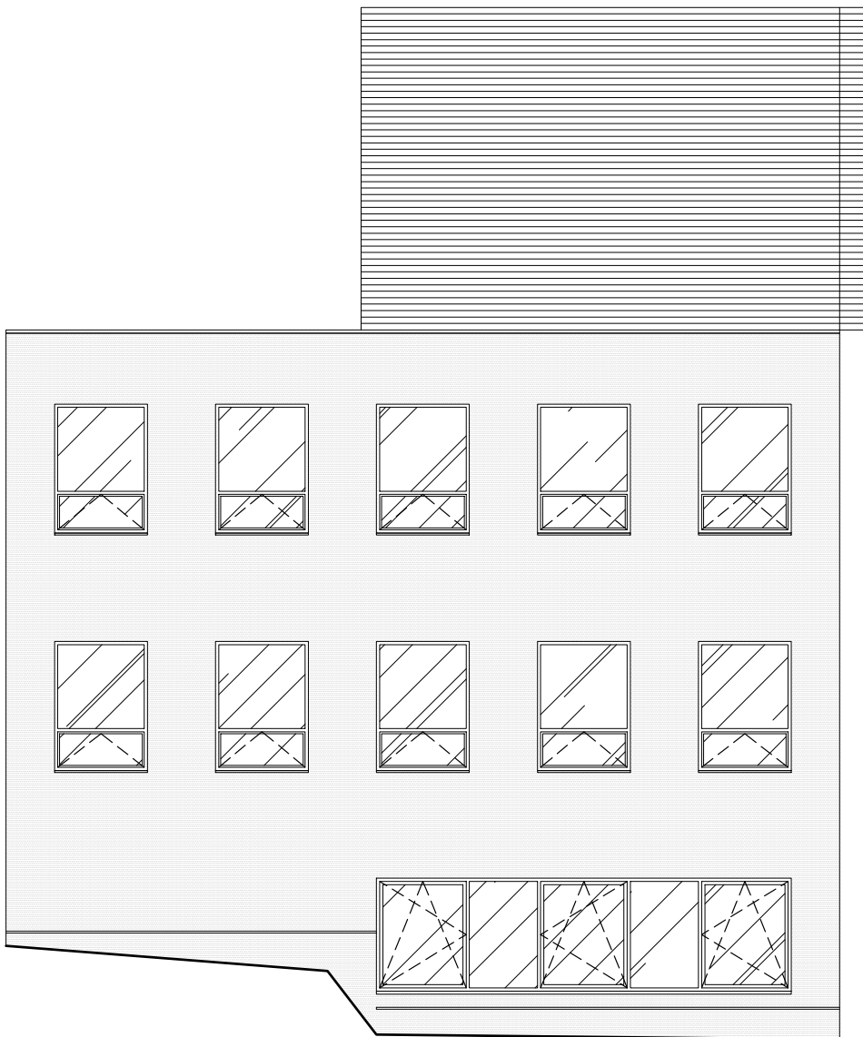
ELEWACJA POŁUDNIOWO - WSCHODNIA (PATIO)
