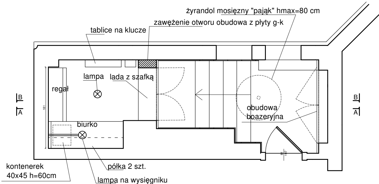
Rzut pomieszczenia recepcji, skala 1:50
