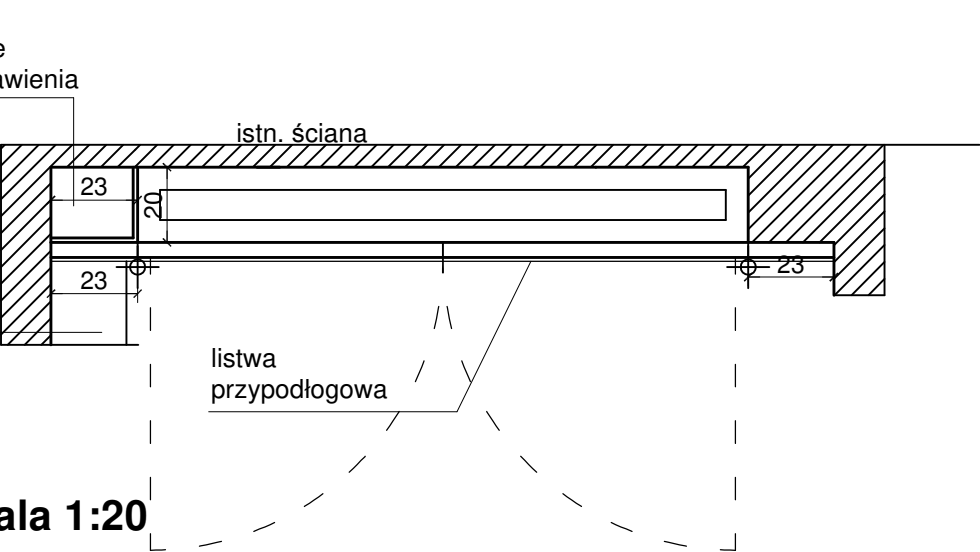
Widok obudowy, skala 1:20
