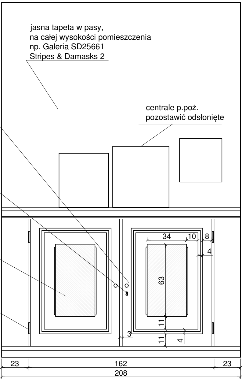
Widok obudowy, skala 1:20
