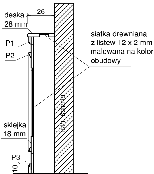
Przekór obudowy, skala 1:20
